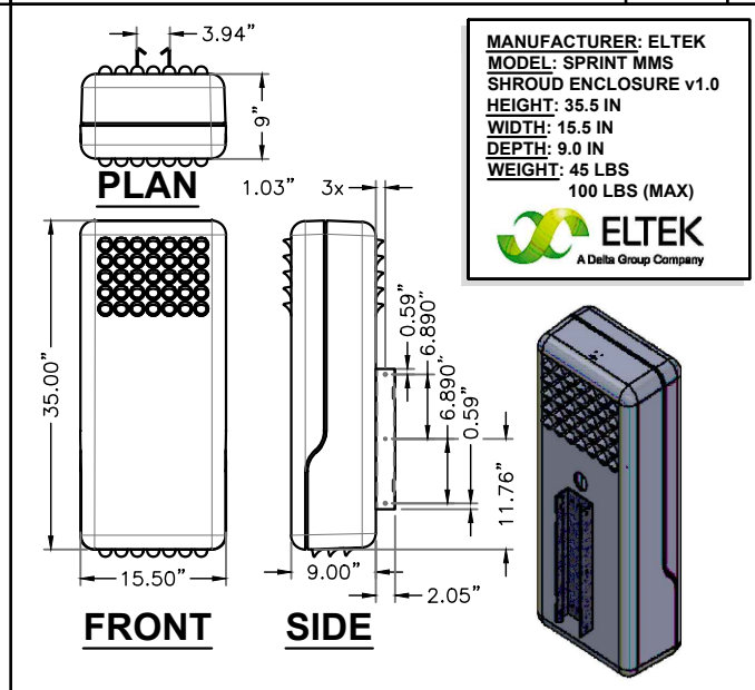
SPRINT MMS SHROUD v1.0 SCALE N.T.S. 6
