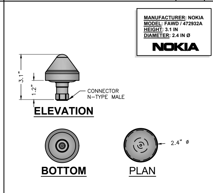
NOKIA GPS UNIT SCALE N.T.S. 9
