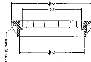
SECTION SCALE N.T.S. A-B DS OF 6
